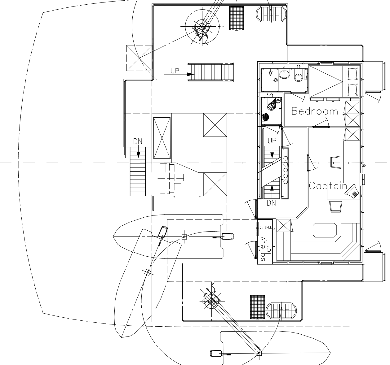
Tween Deck
