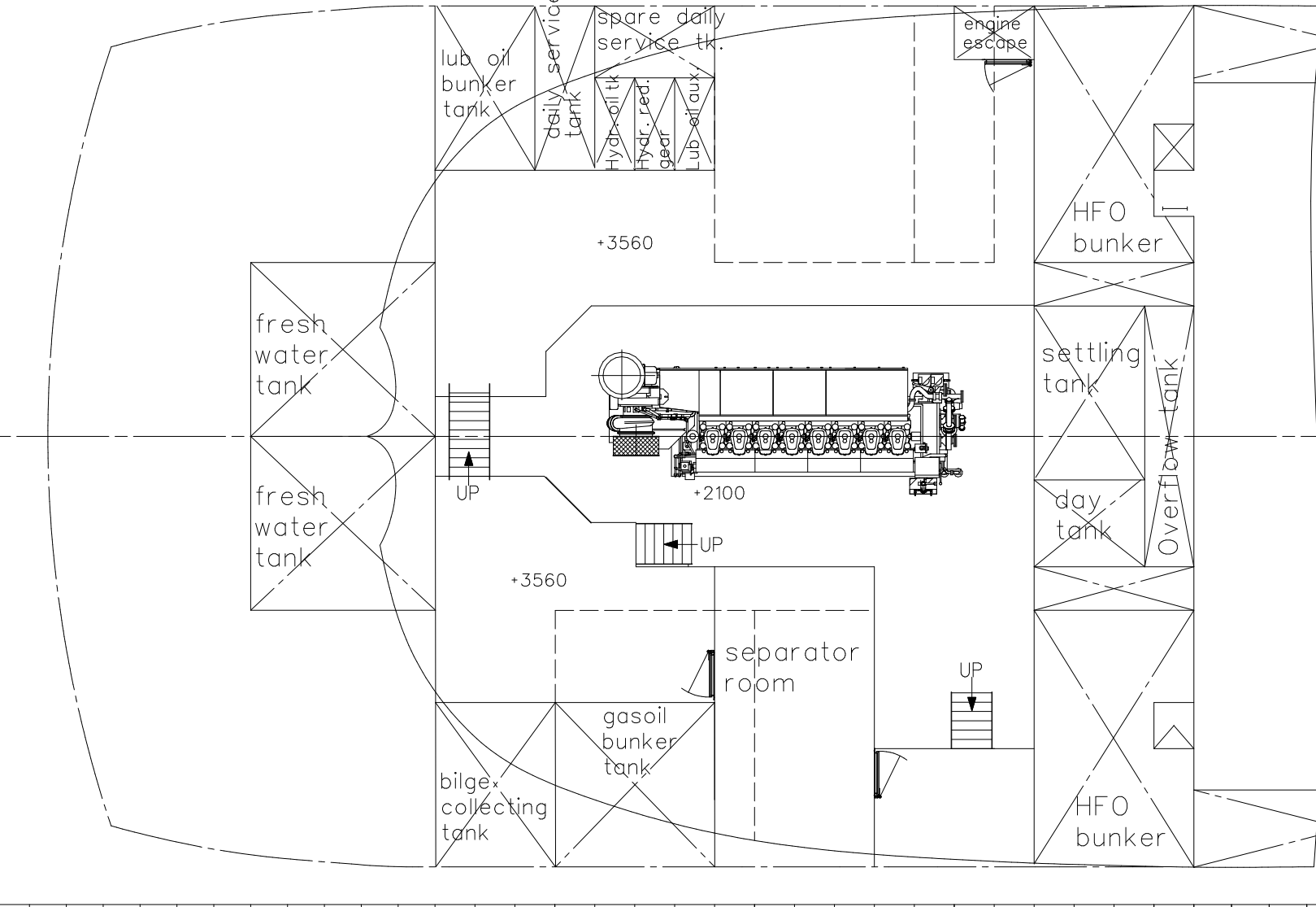
Tween Deck
